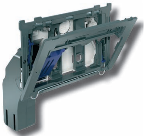
Geberit Blue Plus átszerelő készlet 115.612.00.1
