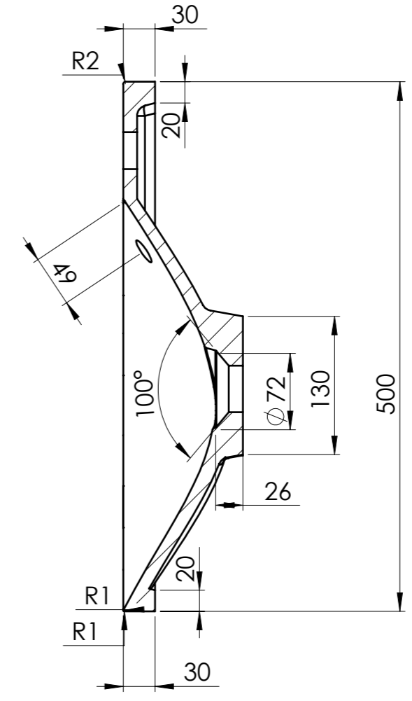
B-B (1 : 5)
