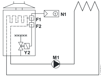
Szobatermosztát falı gázkazán direkt szabályozásával
